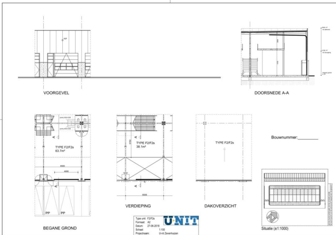
Tekening type F2
