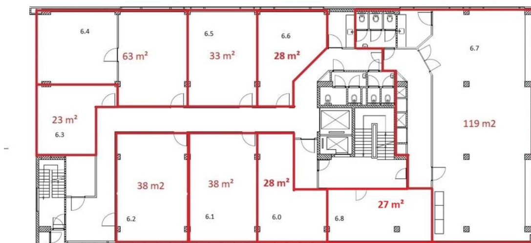
6e verdieping
